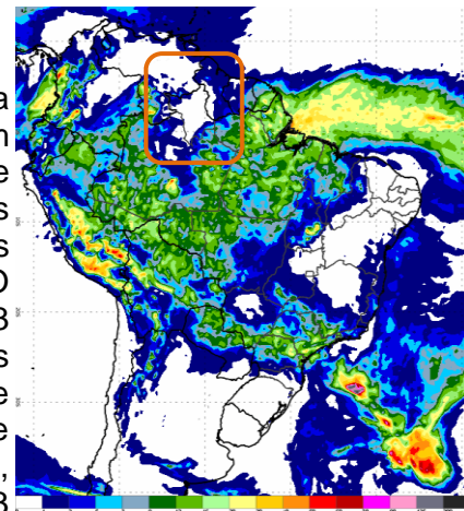
Figura 3 – Modelo de precipitação COSMO (7 x 7km) – INMET
