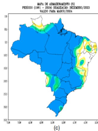
Previsão de armazenamento de água no solo(%) para os meses de (a) janeiro/2024, (b) fevereiro/2024 e (c) março/2024, no Brasil, considerando capacidade de água disponível (CAD) de 100 mm. Fonte: INMET ( https://portal.inmet.gov.br/boletinsagro# )
