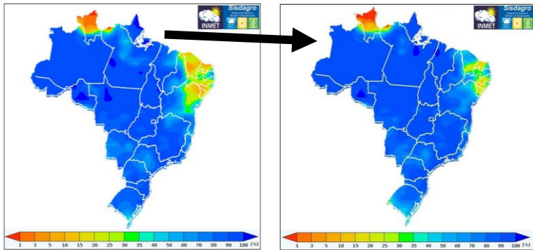
Armazenamento hídrico no solo (%) em janeiro de 2024. Fonte: SISDAGRO/INMET.
