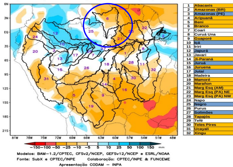
PREVISÃO SUBSAZONAL – MULTIMODELO CALIBRADO Anomalia (mm) de Precipitação Acumulada (14 Dias) Período: 06/03/2024 – 19/03/2024
