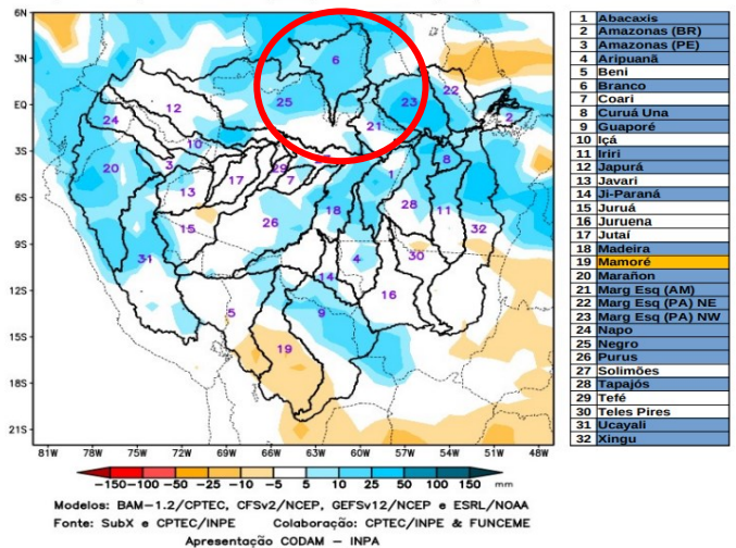
PREVISÃO SUBSAZONAL—MULTIMODELO CALIBRADO Anomalia (mm) de Precipitação Acumulada (07 Dias) Período: 17/04/2024 – 23/04/2024
