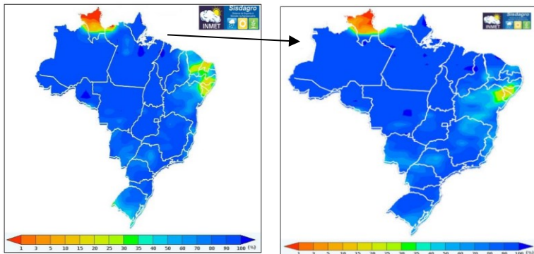
Armazenamento hídrico no solo (%) em fevereiro de 2024. Fonte: SISDAGRO/INMET. Armazenamento hídrico no solo (%) em março de 2024. Fonte: SISDAGRO/INMET.
