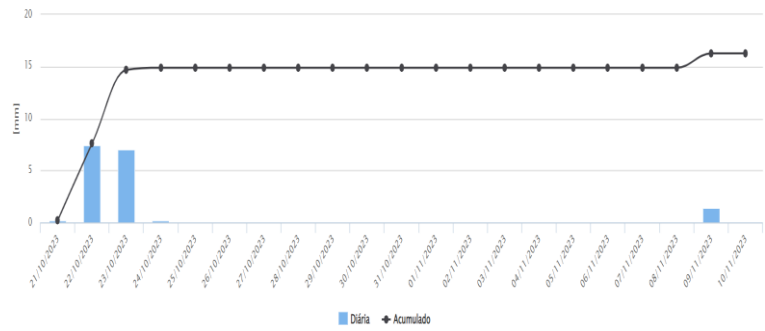
Estação: Olímpico (140010004A) | Tipo: Pluviométrica | Município: BOA VISTA/RR | Fonte: CEMADEN
