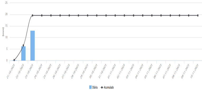
Estação: Calunga (140010002A) | Tipo: Pluviométrica | Município: BOA VISTA/RR | Fonte: CEMADEN
