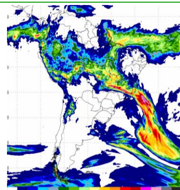
Figura 2 - Modelo COSMO (7 x 7km) - INMET. Modelo de precipitação acumulada para 26/1/2020
