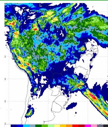
Figura 2 - Modelo COSMO (7 x 7km) - INMET. Modelo de precipitação acumulada para 1/1/2021
