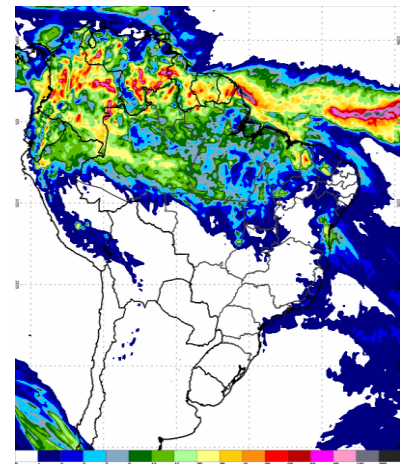
Figura 3 – Modelo de precipitação COSMO (7 x 7km) – INMET para dia 30/04/2021
